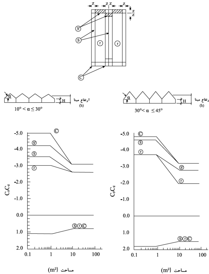
شکل ۳-۱۳ - ضرایب فشار خارجی C_{pe}C_{eg} در سقف‌های شیروانی چند دهانه با شیب بزرگ‌تر از 10^\circ
