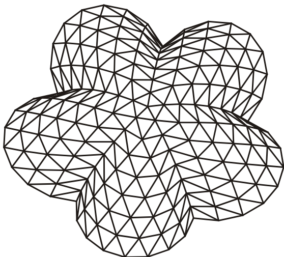
شکل ۱۱۴- گنبد اسکالپ با کد ۱، برآمدگی ۸ و پیش‌آمدگی ۱۵
