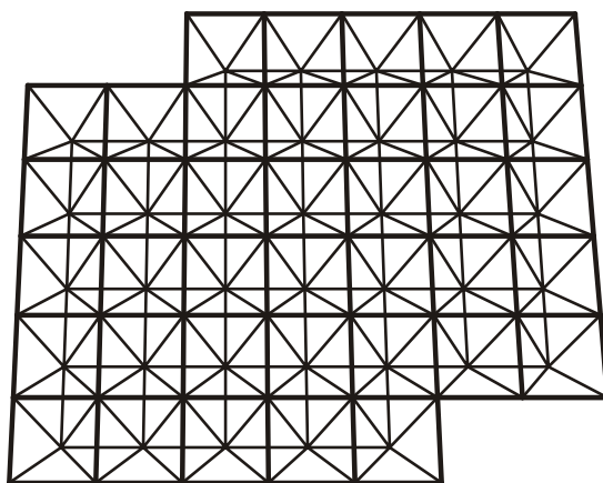
شکل ۶۵- شبکه دو لایه مرکب با نقش دوراهه روی دوراهه
