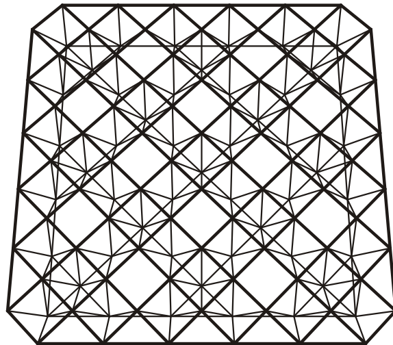
شکل ۴۴ - شبکه دو لایه با نقش اریبی روی اریبی بزرگتر
