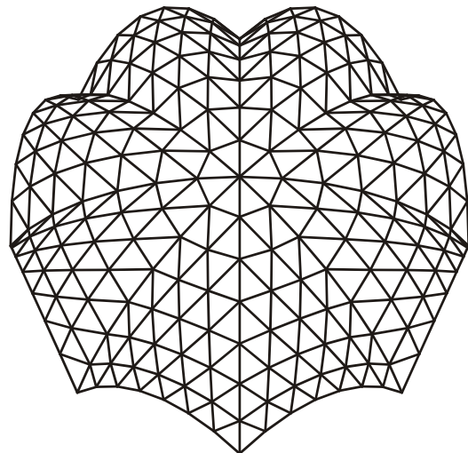
شکل ۱۱۳- گنبد اسکالپ با کد ۱، برآمدگی ۱۵ و پیش‌آمدگی صفر
