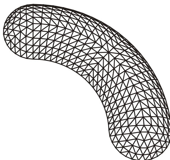
شکل ۱۶۴ - چلیک - گنبد پهلوخمیده
