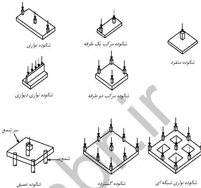
شکل ۹-۱۵-۱ انواع شالوده‌ها
