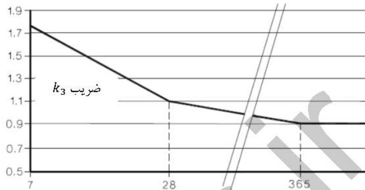
شکل ۹-۴-۱ ضریب k_3
