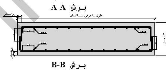
شکل ۹-۶-۹ مشخصات پی ساختمان
