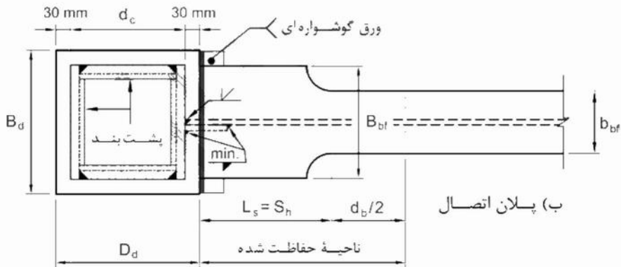
شکل ۳-۱۰-۷-۱۵: گزینه دیگر برای اتصال گیردار تیر با بال پهن شده و دیافراگم عبوری از ستون
