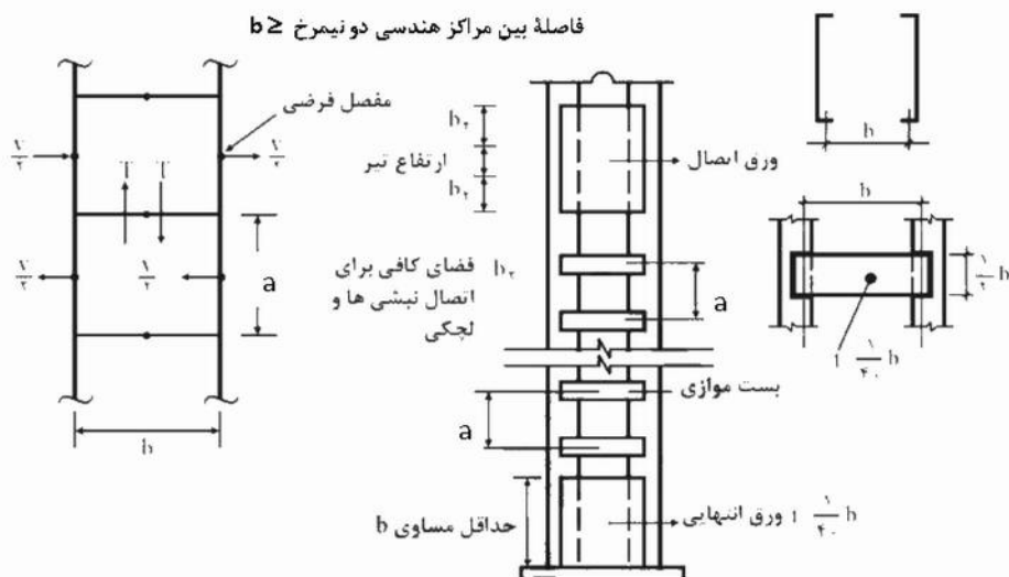
شکل ۱۰-۲-۴-۴: عضو فشاری ساخته شده (مکعب) با بست‌های موازی
