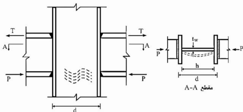
شکل ۱۰-۲-۹-۲۷: کمانش فشاری جان در مقابل یک جفت نیروی متمرکز فشاری
