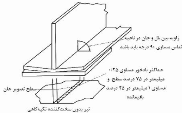
شکل ۱۵-۴-۱۰: رواداری در محل تماس تیر با تکیه‌گاه - تیر بدون سخت‌کننده تکیه‌گاهی
