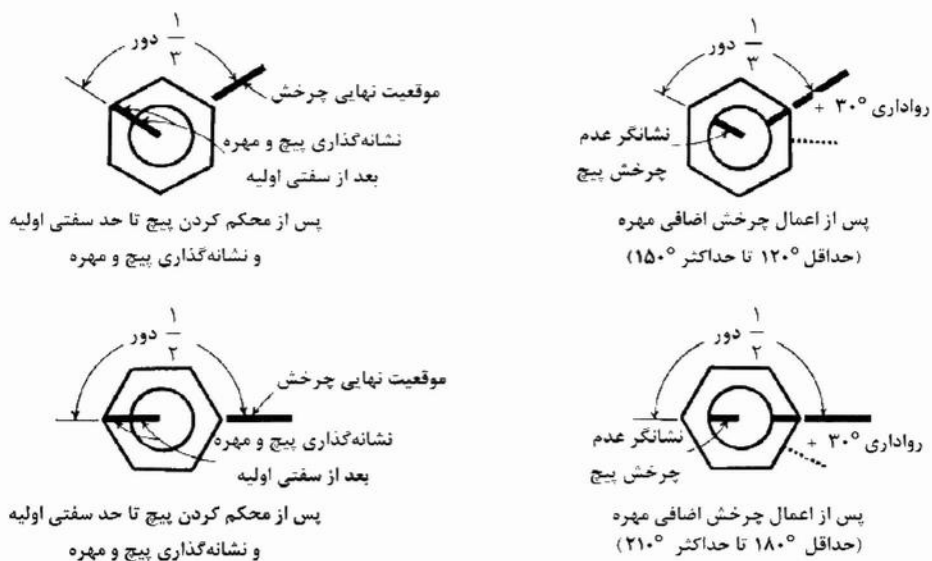
شکل ۴-۱۰-۴: دستورالعمل چرخش مهره
