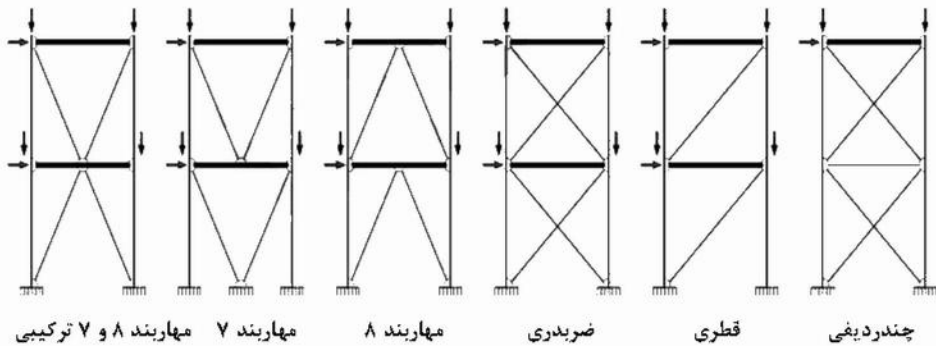
شکل ۱-۱-۴-۳-۱۰: چند نمونه مجاز از پیکربندی مهاربندهای همگرا
