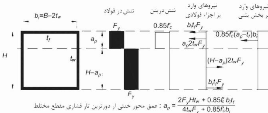
شکل ۱۰-۲-۸-۱۳: محاسبه لنگر خمشی پلاستیک مقطع مختلط پر شده با بتن برای مقاطع فشرده
