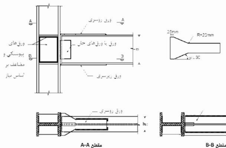
شکل ۳-۱۰-۶: اتصال گیردار جوشی به کمک ورق‌های روسری و زیرسری (WFP)
