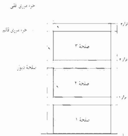
شکل ۱۰-۳-۴-۵-۱: پی‌کربندی دیوار برشی فولادی ویژه
