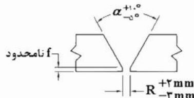
(پ) جوش شیاری بدون پشت‌بند-با جوش پشت
