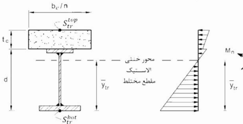
شکل ۱۰-۳-۸-۴: توزیع الاستیک تنش در مقطع مختلط تبدیل‌یافته در صورت استفاده از پایه‌های موقت
