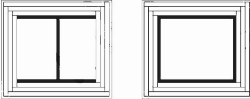
شکل ۱۰-۶-۲: حفاظت ستون‌های فولادی با استفاده از گچ برگ‌ها
