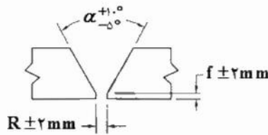
(الف) جوش شیاری بدون پشت‌بند-بدون جوش پشت
