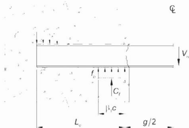
شکل ۱۰-۳-۶-۳-۱: طول آزاد و طول مدفون تیر همبند
