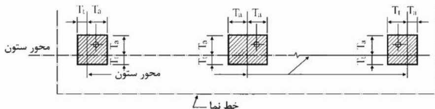
شکل ۱۰-۴-۱۸: ناراستایی ستون‌های داخلی
