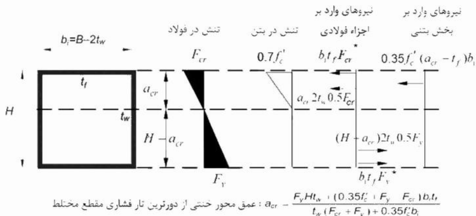
شکل ۱۰-۲-۸-۱۵: محاسبهٔ لنگر خمشی مقطع مختلط در صورتی که مقطع فولادی دارای اجزای لاغر باشد
