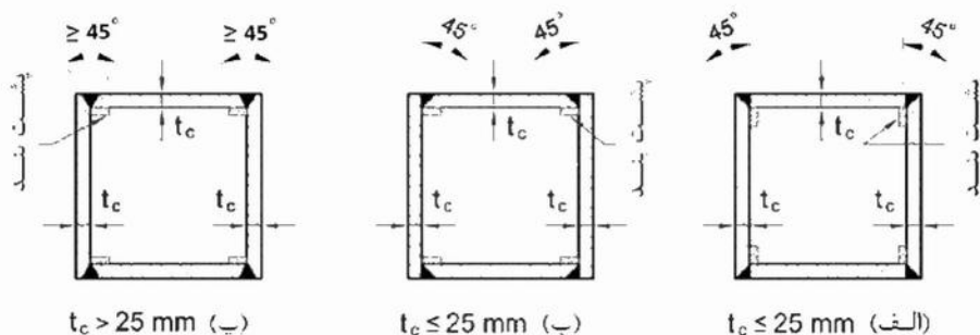
شکل ۱۰-۳-۷-۱: نحوه ساخت ستون‌های جعبه‌ای ساخته شده از ورق
