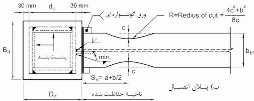
شکل ۱۰-۳-۷-۱۰: اتصال گیردار تیر با مقطع کاهش یافته و دیافراگم عبوری از ستون (TD-RBS)
